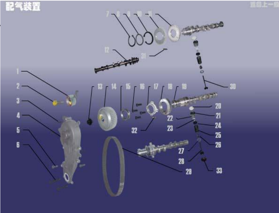
E-17 配气装置---AIR DISTRIBUTING DEVICE
